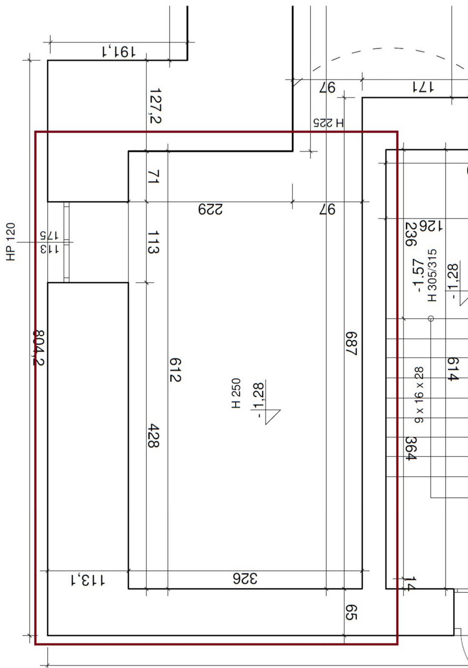
Rys. 1 Pomieszczenie szubienicy
