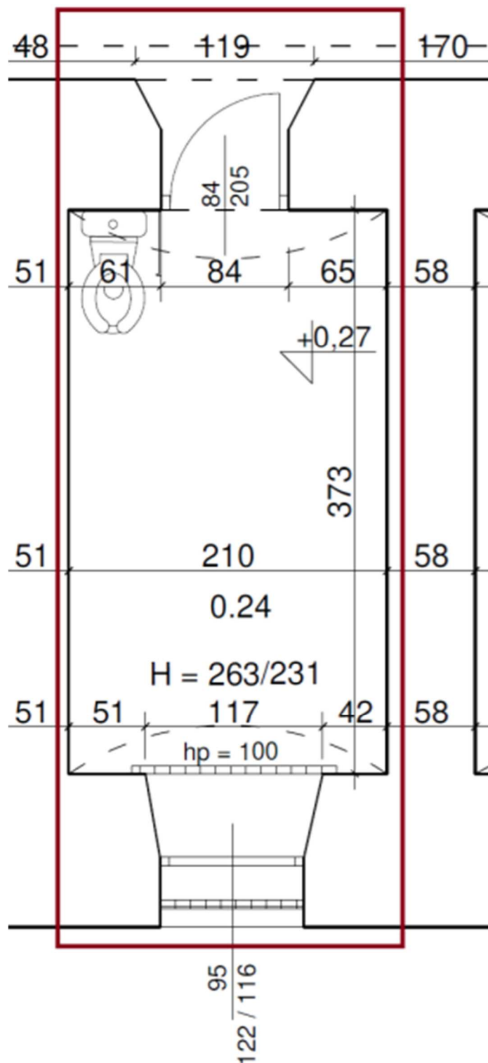
Rys. 3 Cela nr 6
